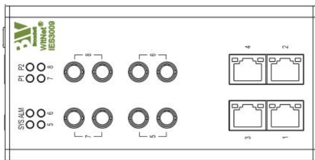
图 3-2 WitNet IES3009 前面板图
