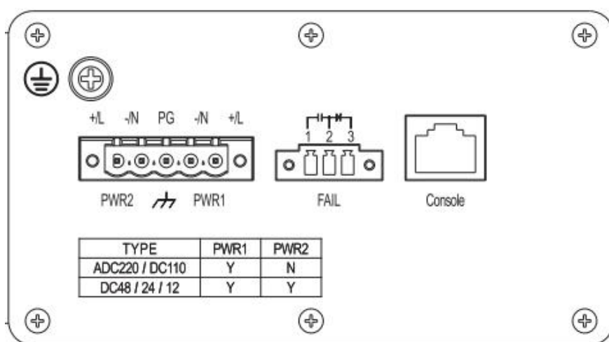
图 3-3 WitNet IES3009 上面板图
