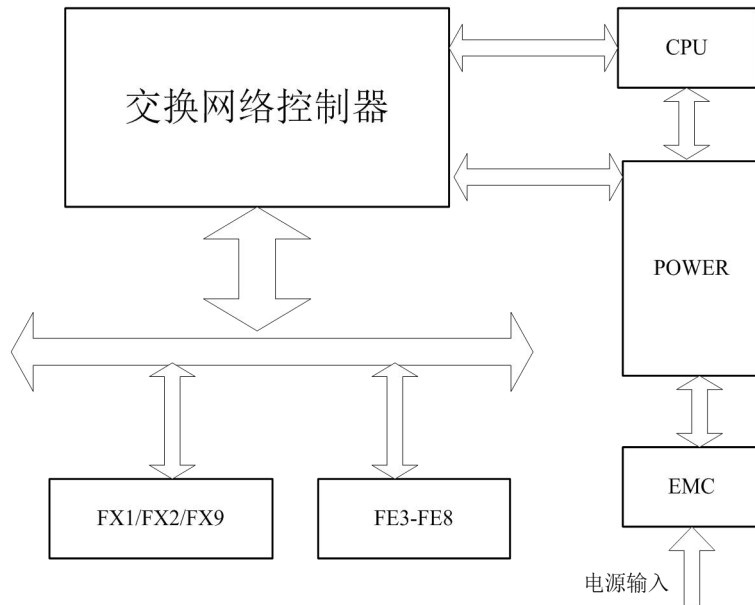
图 3-1 WitNet IES3009 硬件结构图
