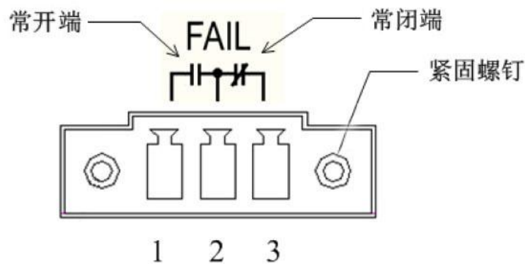
图 3-6 告警端子
