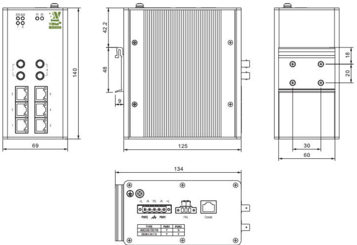
图 4-2 WitNet IES3009 安装尺寸图
